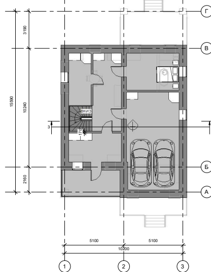
План 2 этажа
