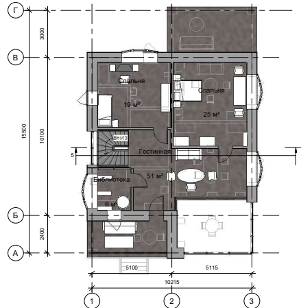
План 2 этажа
