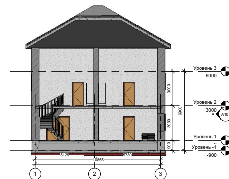
Северный фасад
