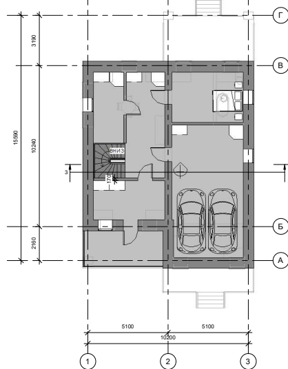
план 2 этажа
