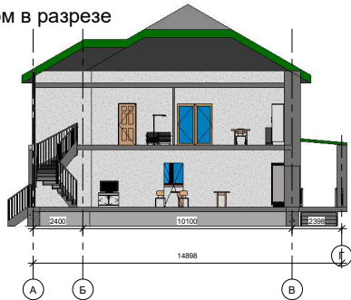
дом в разрезе
