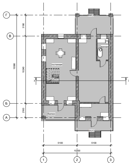
План 1 этажа
