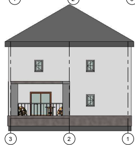
Северный фасад
