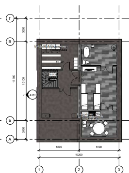
ПЛАН -1 ЭТАЖА
