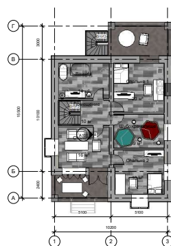
ПЛАН 2 ЭТАЖА
